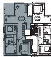
VERDIEPINGSPLAN
